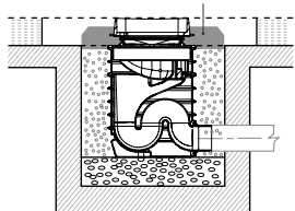
6 anello di supporto della griglia in cemento
