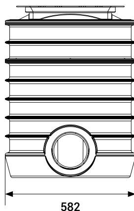
vista frontale, uscita sifone
