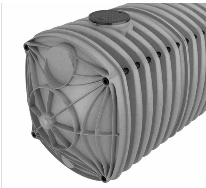
Particolare della vista frontale. Geometria progettata per grossi carichi del terreno.
