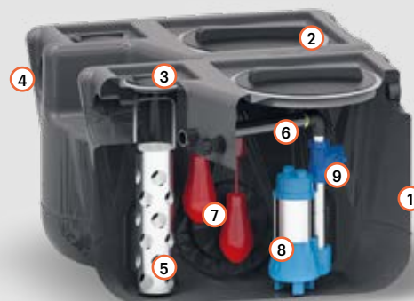
DOPPIA VASCA
