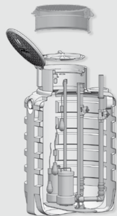
SOL CC CON POMPA E PIEDE D'ACCOPPIAMENTO
